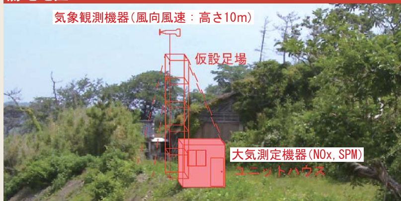
大気観測機器設置例(風向風速、ユニットハウス)
